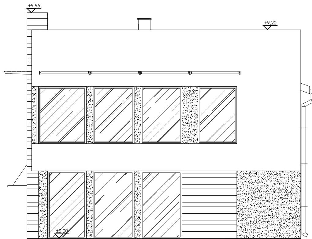
ELEWACJA PÓŁNOCNA
